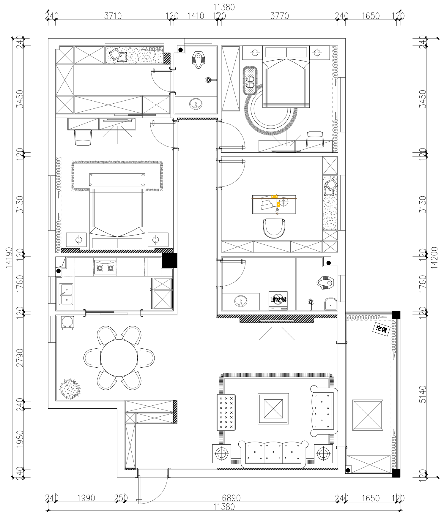
平面布局图 1:100
